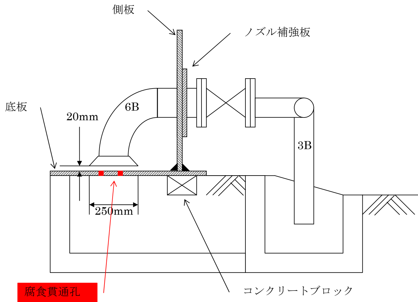
図 ドレンノズルの構造
