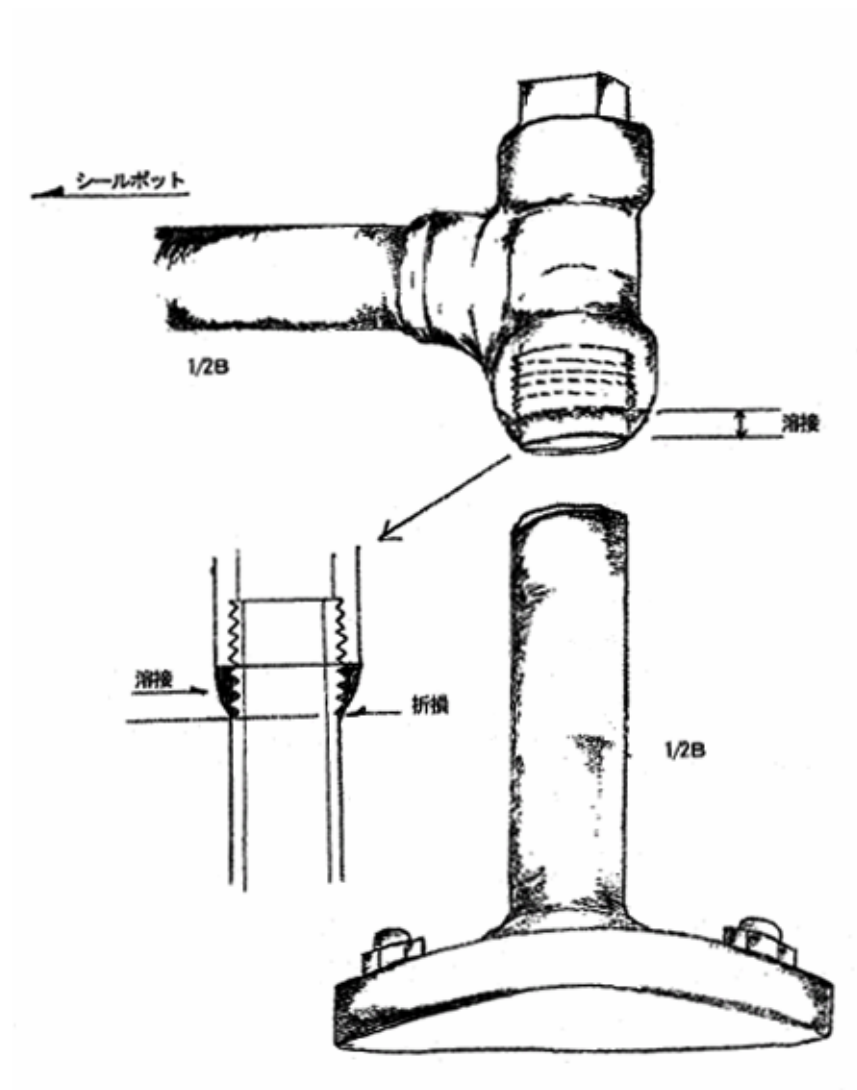
図 折損箇所の詳細
