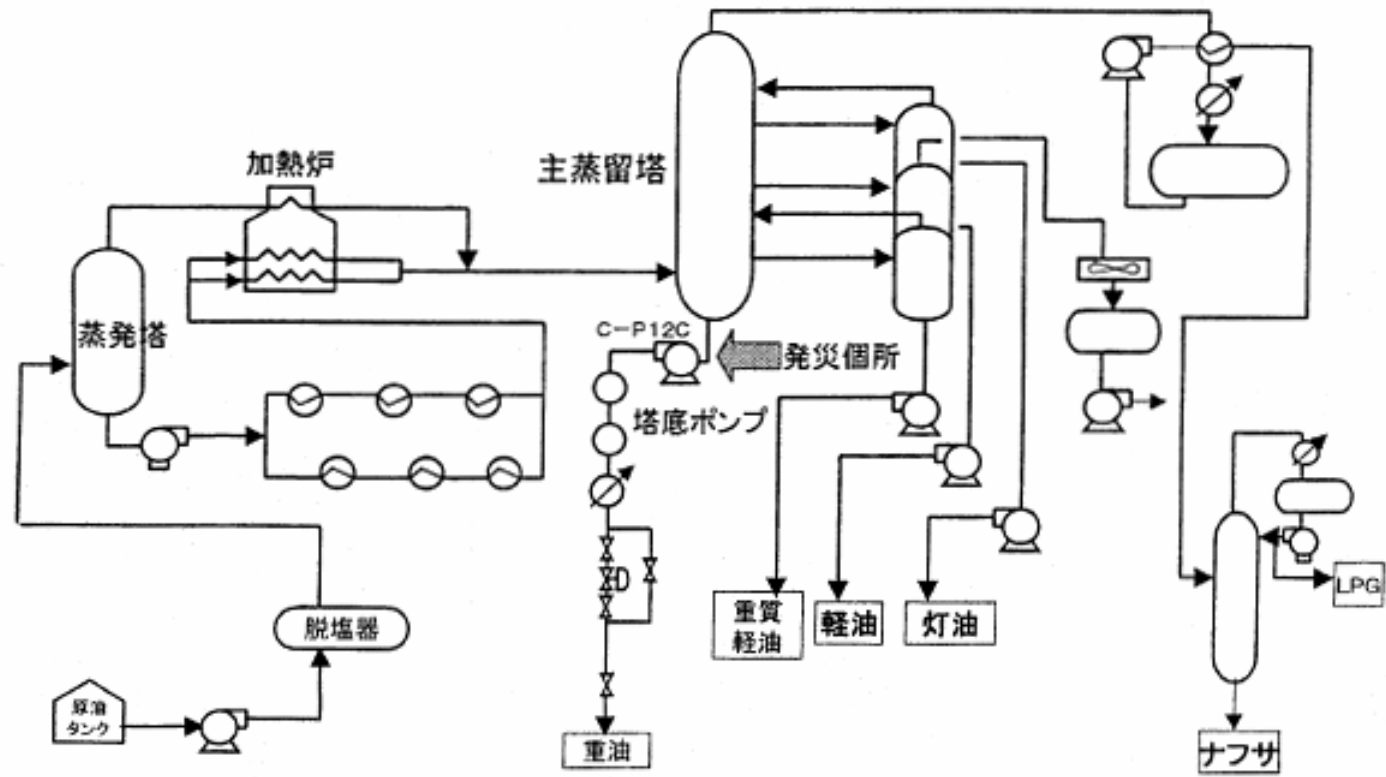
図 常圧蒸留装置概略フロー
