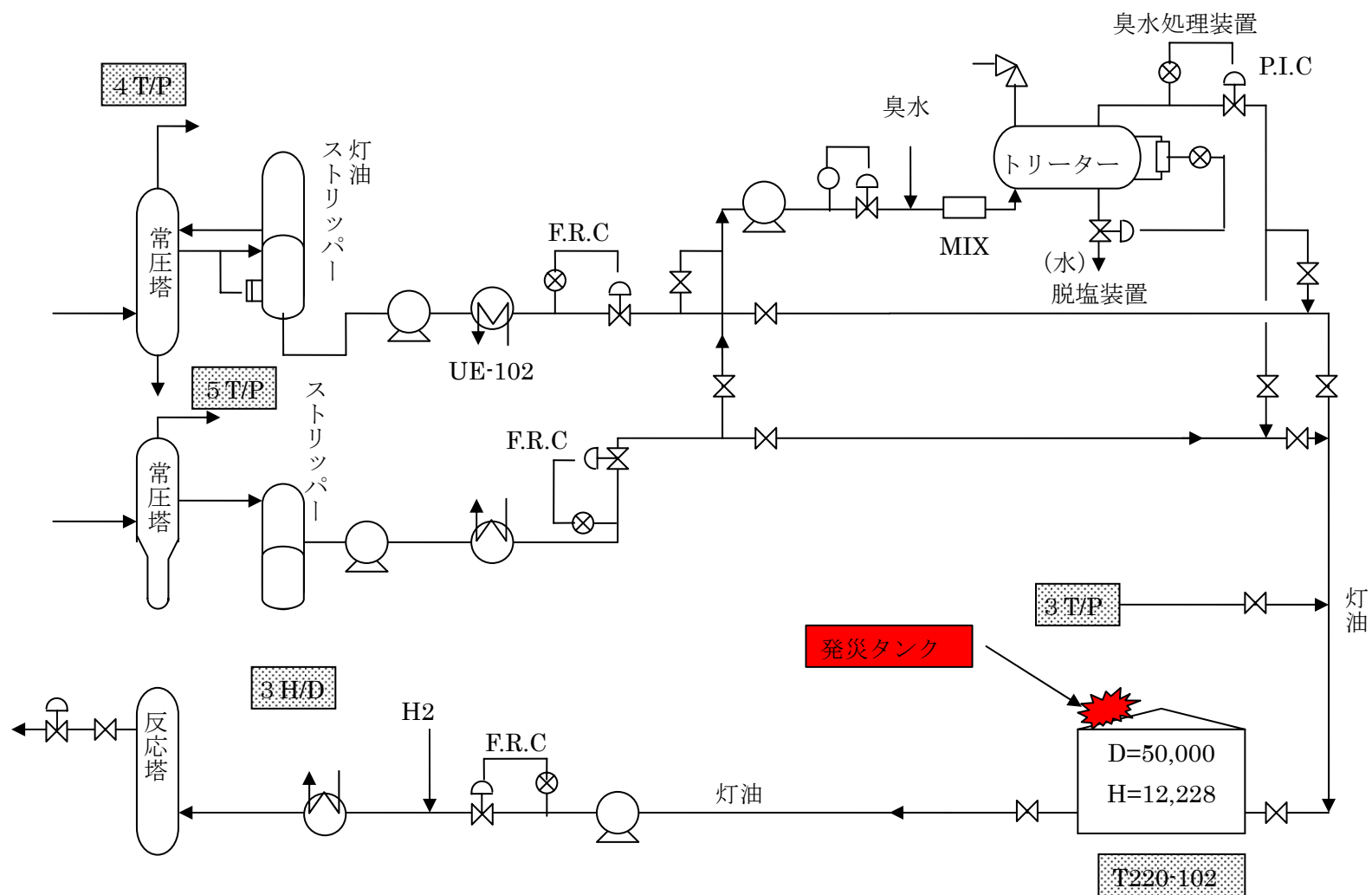
図 プロセス及び設備の概要
