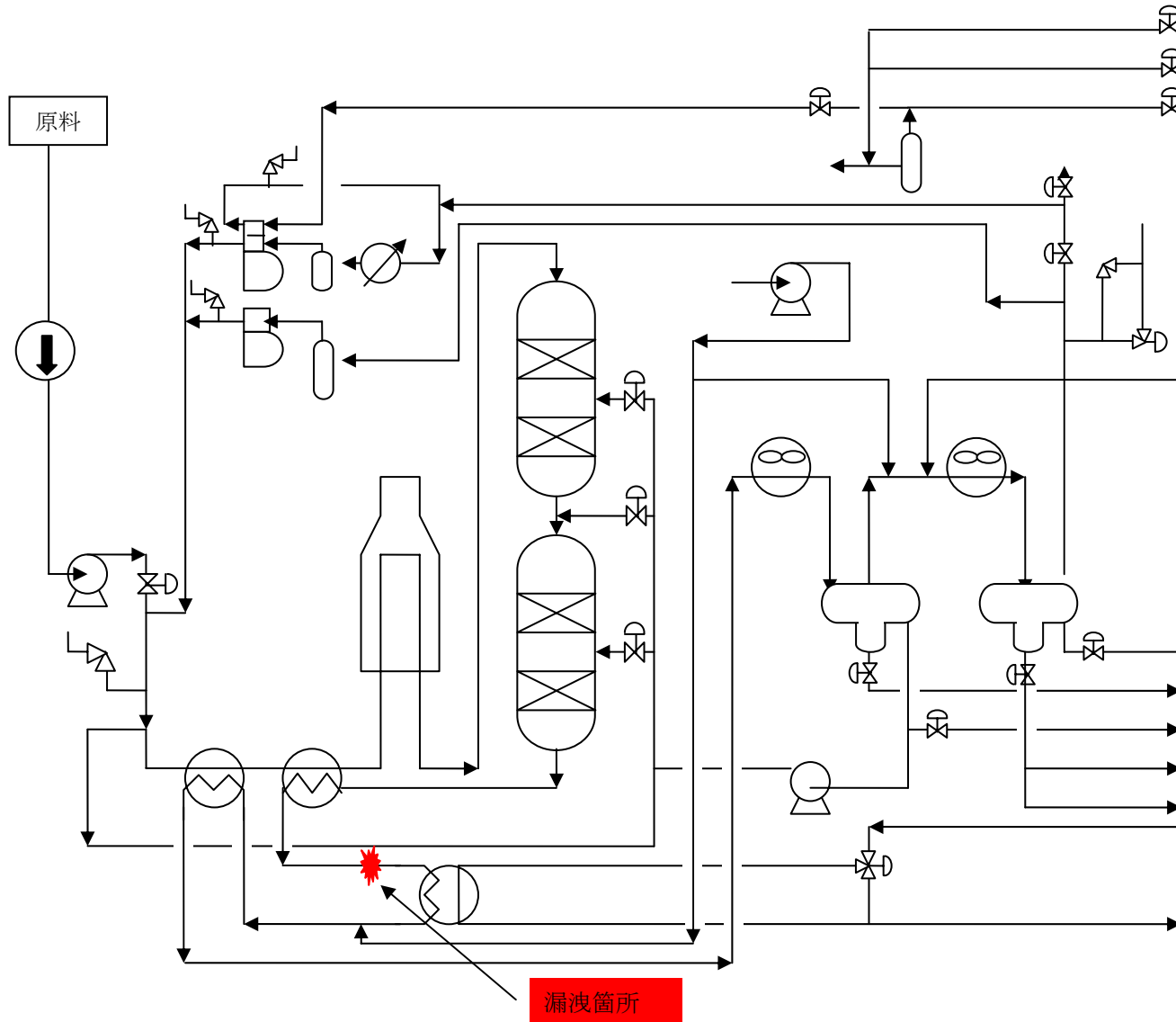
図1 水素化脱硫装置プロセスフロー
