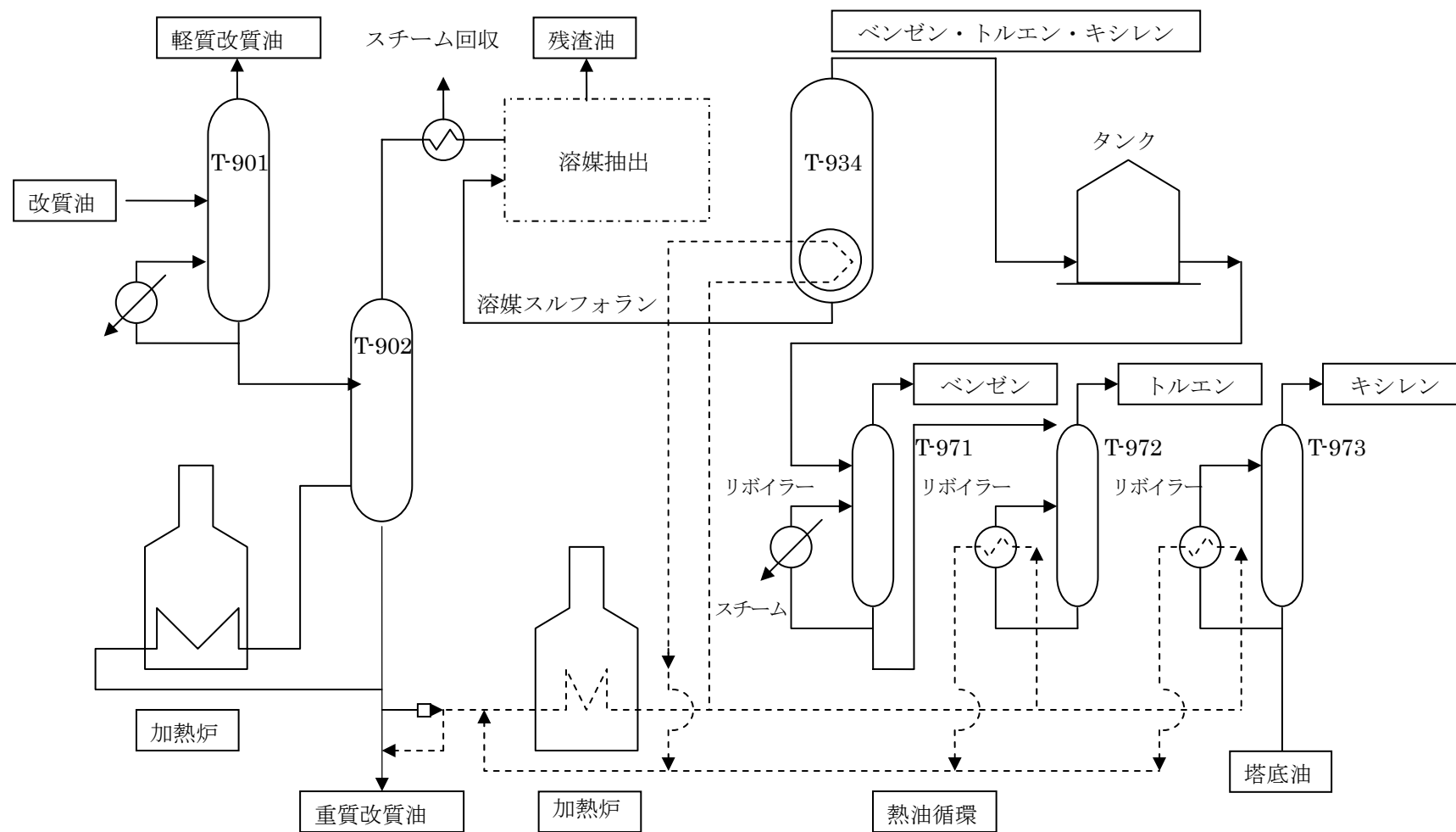
図 BTX 装置工程図
