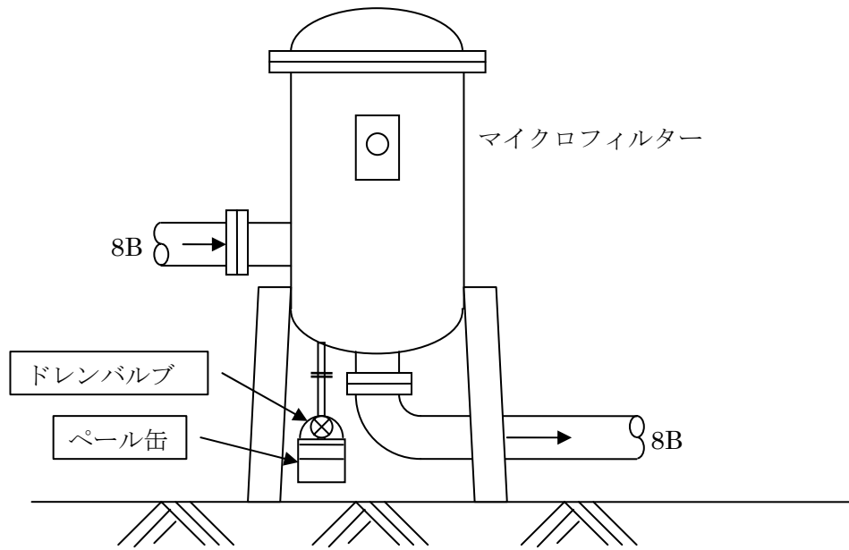
図 設備概略図
