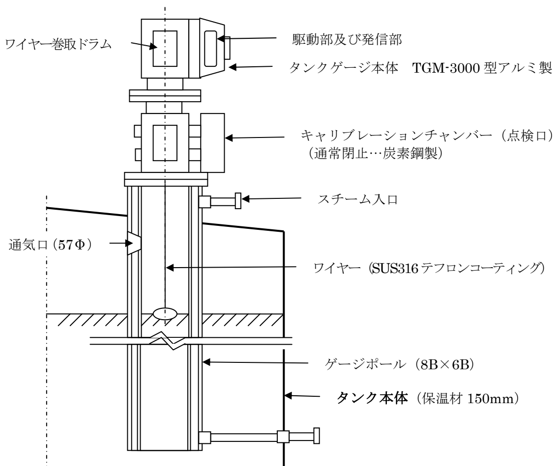
図 2 液面計取付状況図
