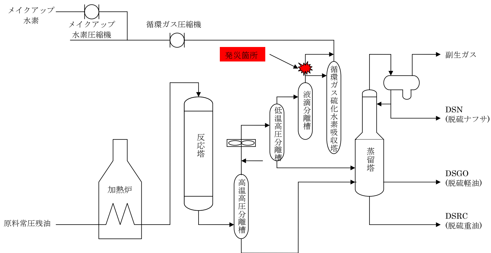
図1 重油直接脱硫装置フローと破損箇所
