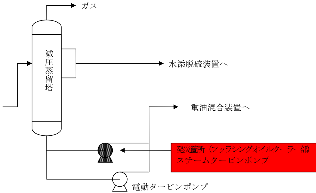
図1 減圧蒸留塔付近のフロー
