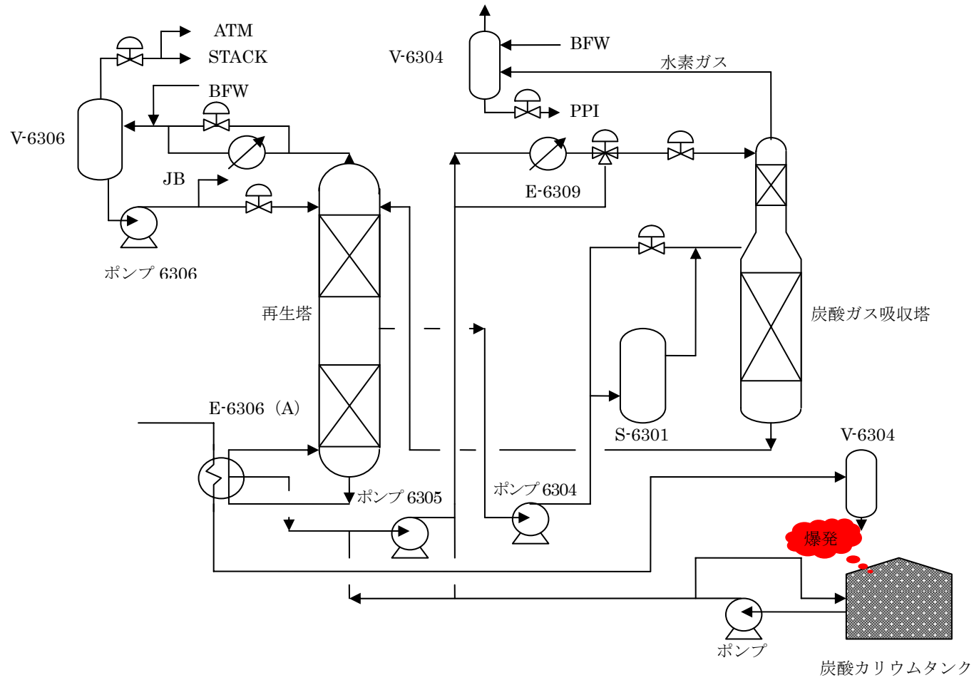
図 炭酸カリウム水溶液の回収タンク付近のフロー
