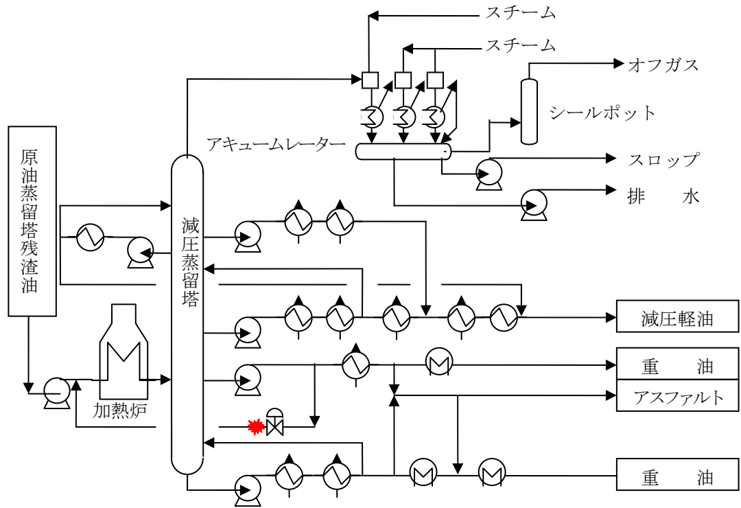
図1 減圧蒸留装置概略工程図
