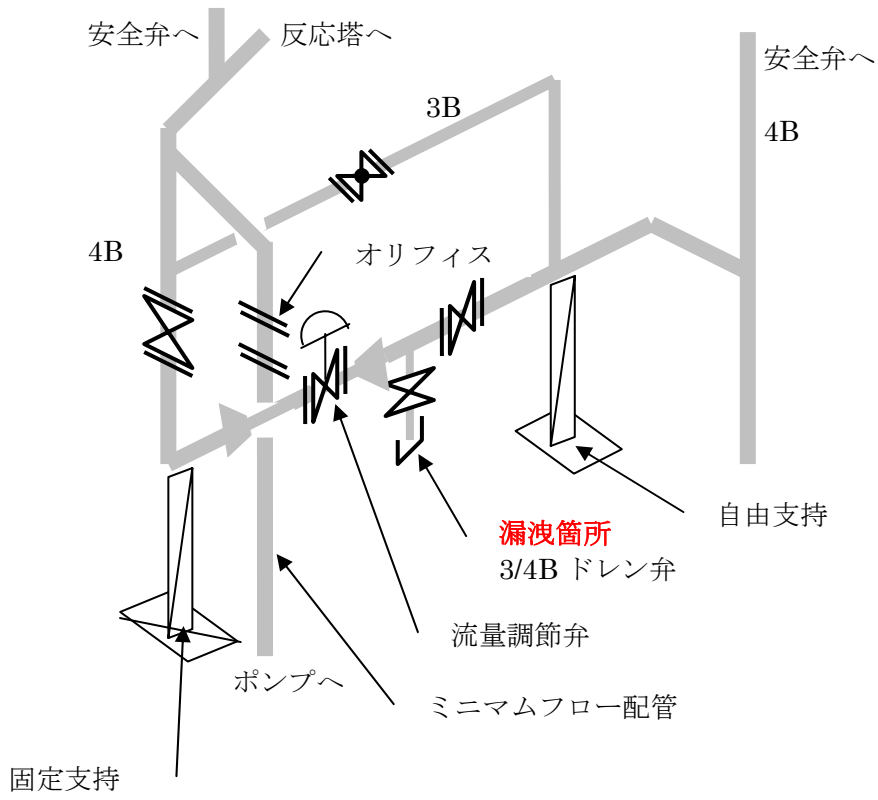
図 流量調節弁まわりの配管図
