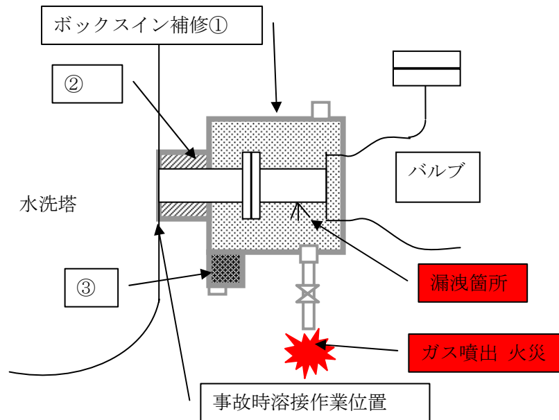
図 2 ボックスイン補修図
