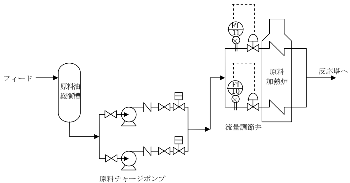
図 重油脱硫装置のフロー
