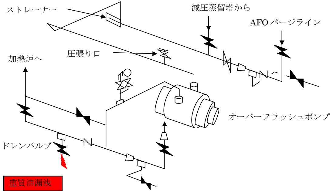
図2 オーバーフラッシュポンプ周辺配管図
