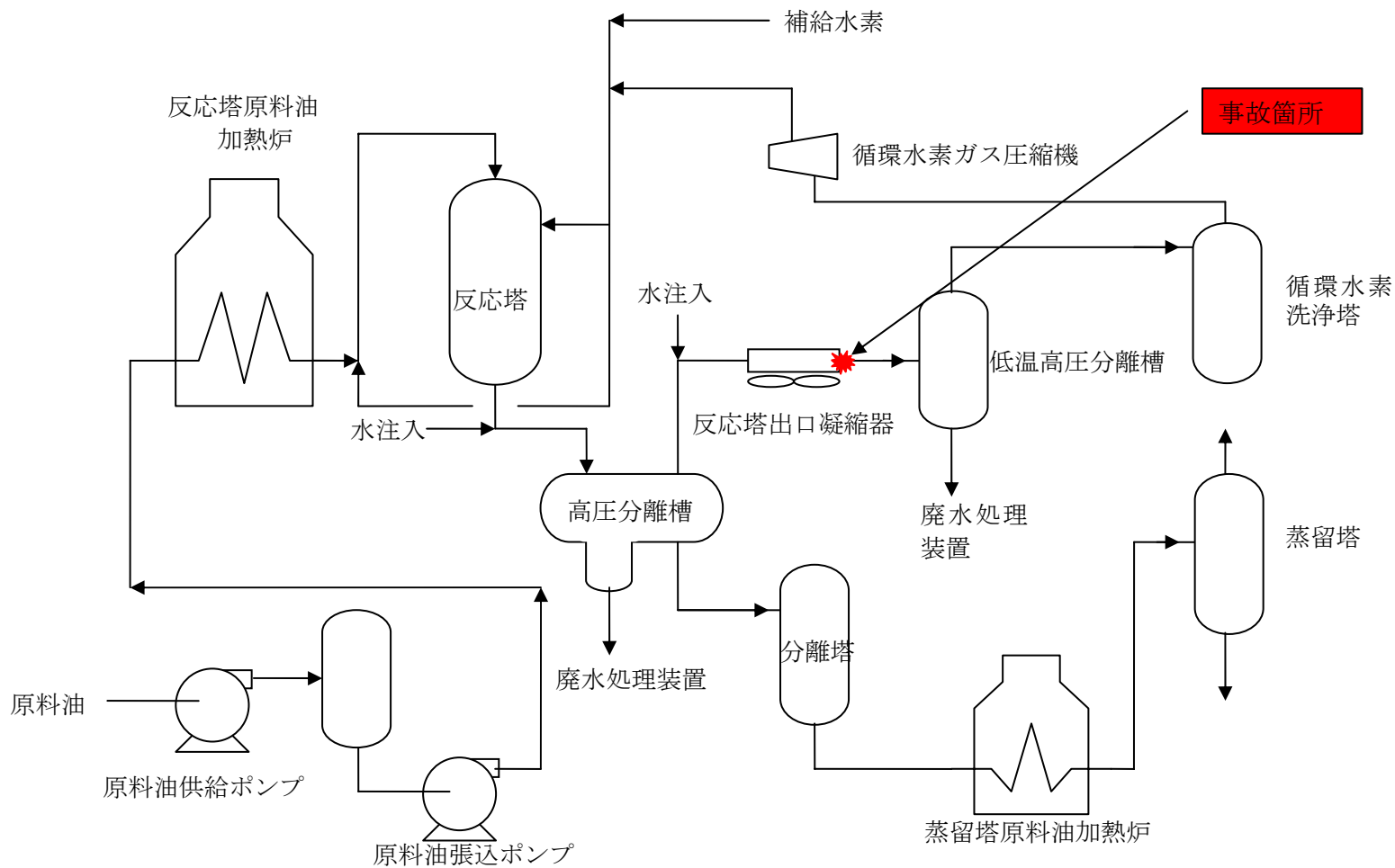
図1 重油間接脱硫装置フロー図
