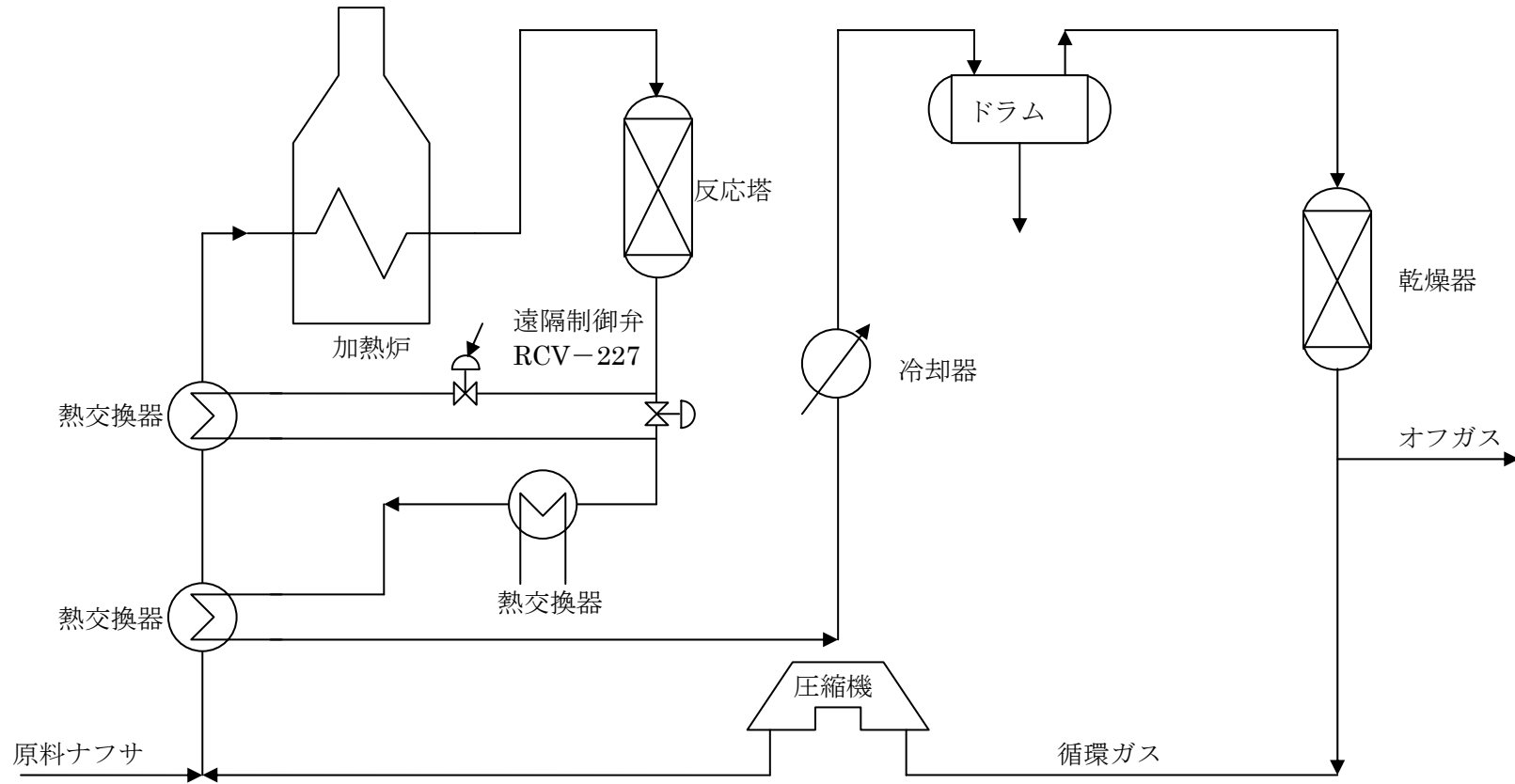
図 接触改質装置概略工程図
