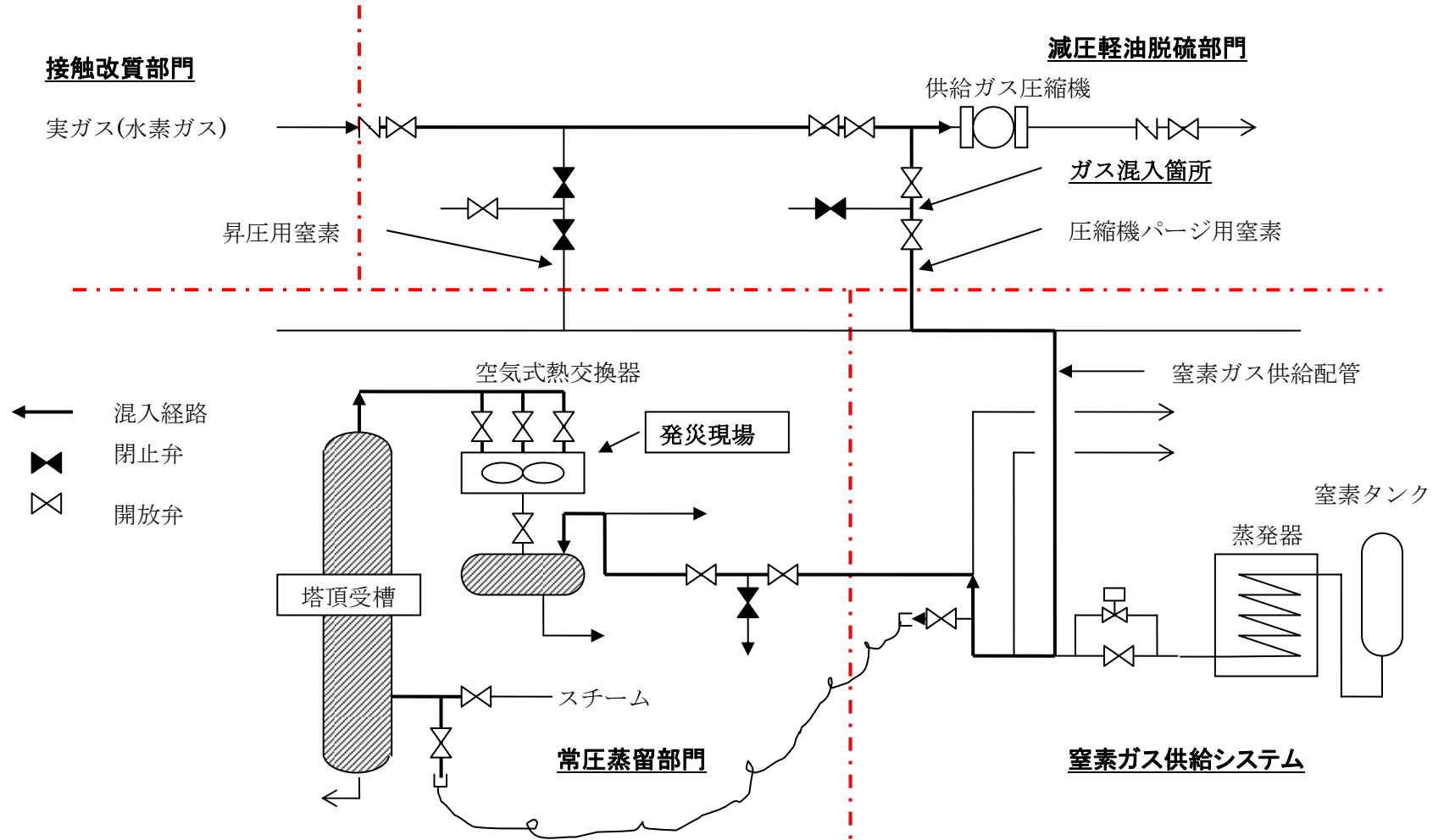
図2 窒素供給配管への実ガス混入経路
