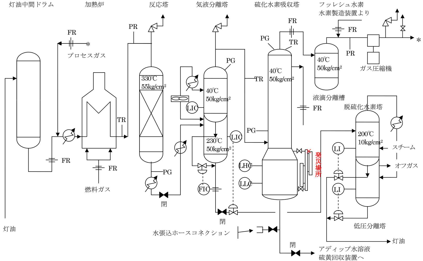
図 水添脱硫装置フローシート
