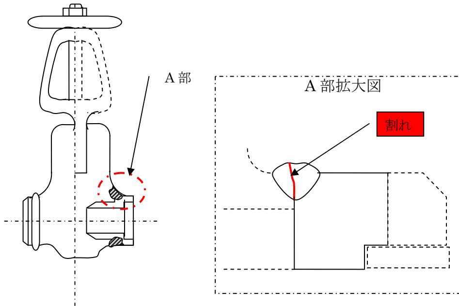
図2 バルブ破損状況
