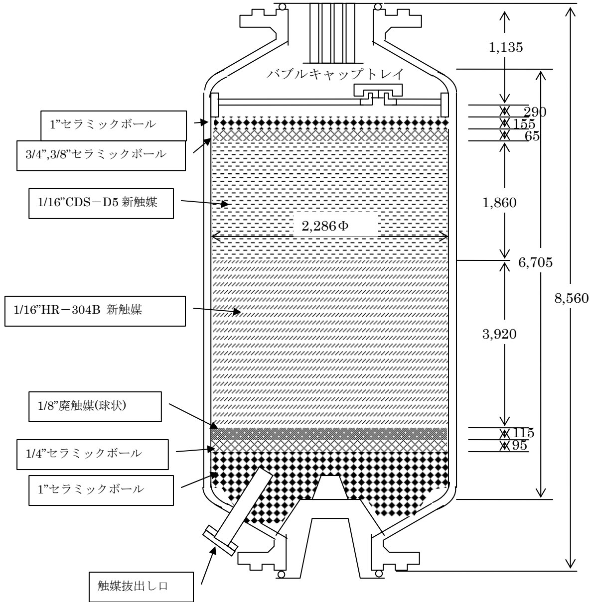
図2 反応塔・触媒充填構造図
