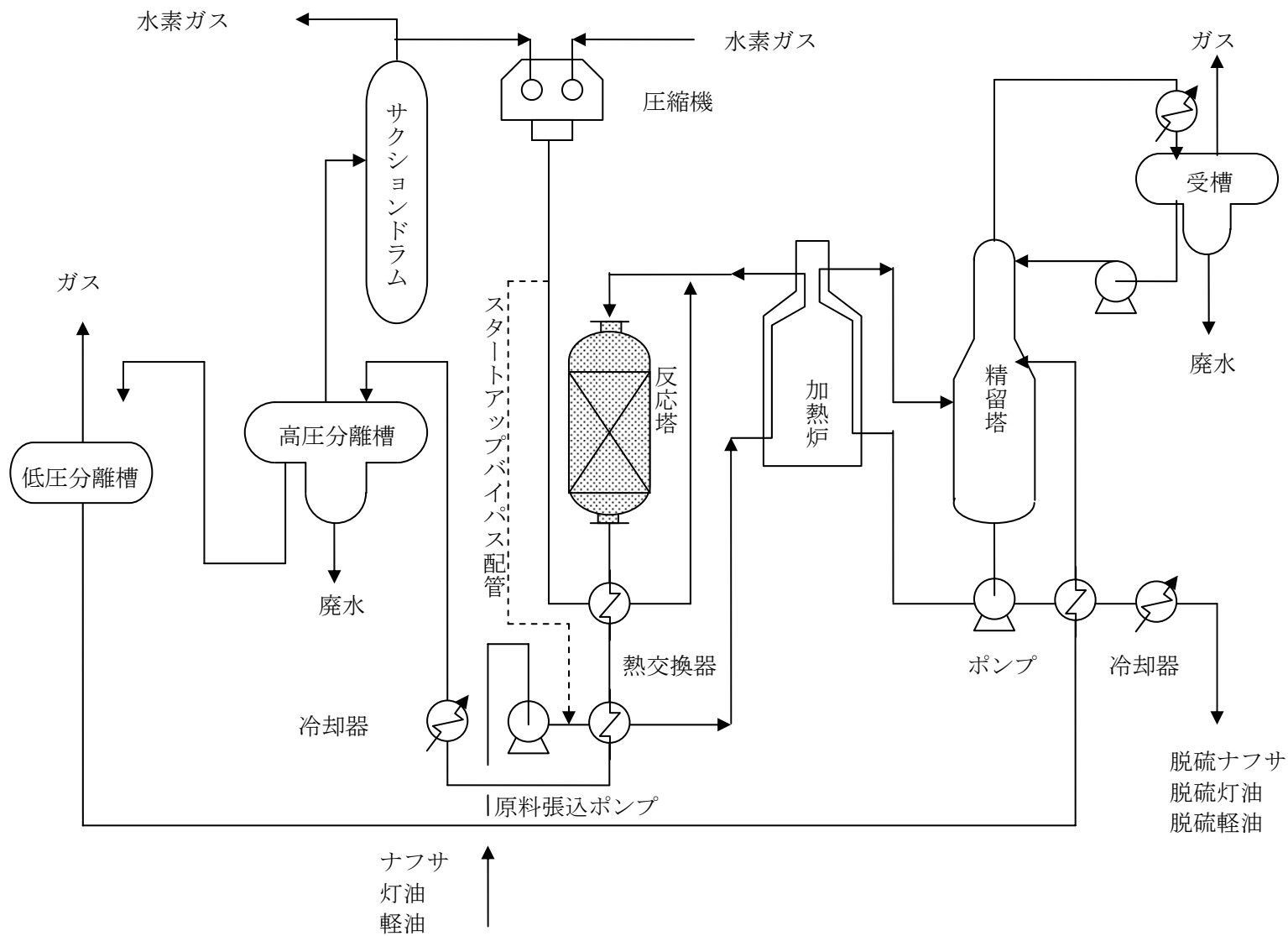
図1 水添脱硫装置フローシート
