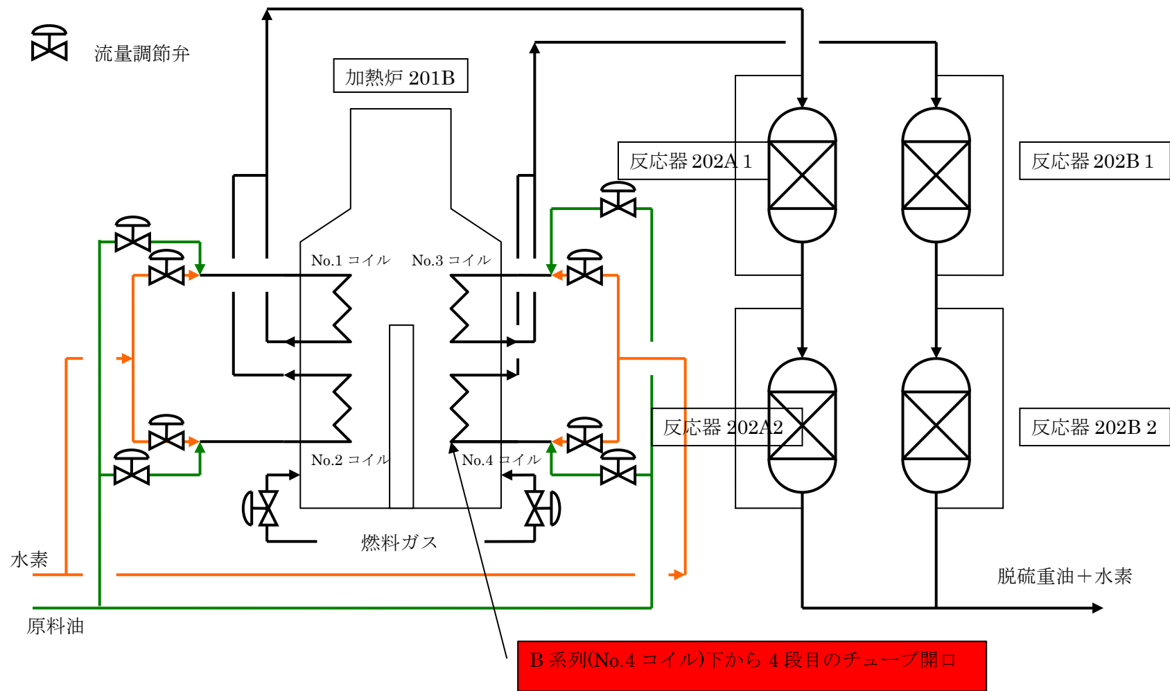
図 重油脱硫装置加熱炉廻りフロー
