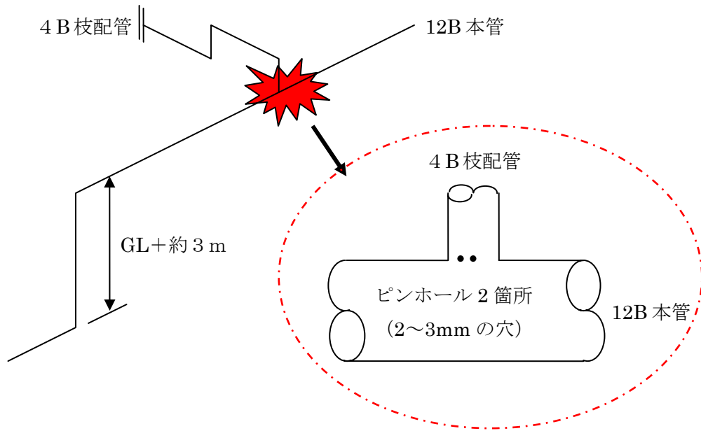
図 C 重油移送配管漏洩箇所
