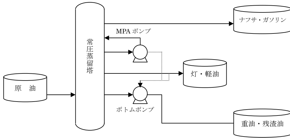
図1 設備・機器の概要
