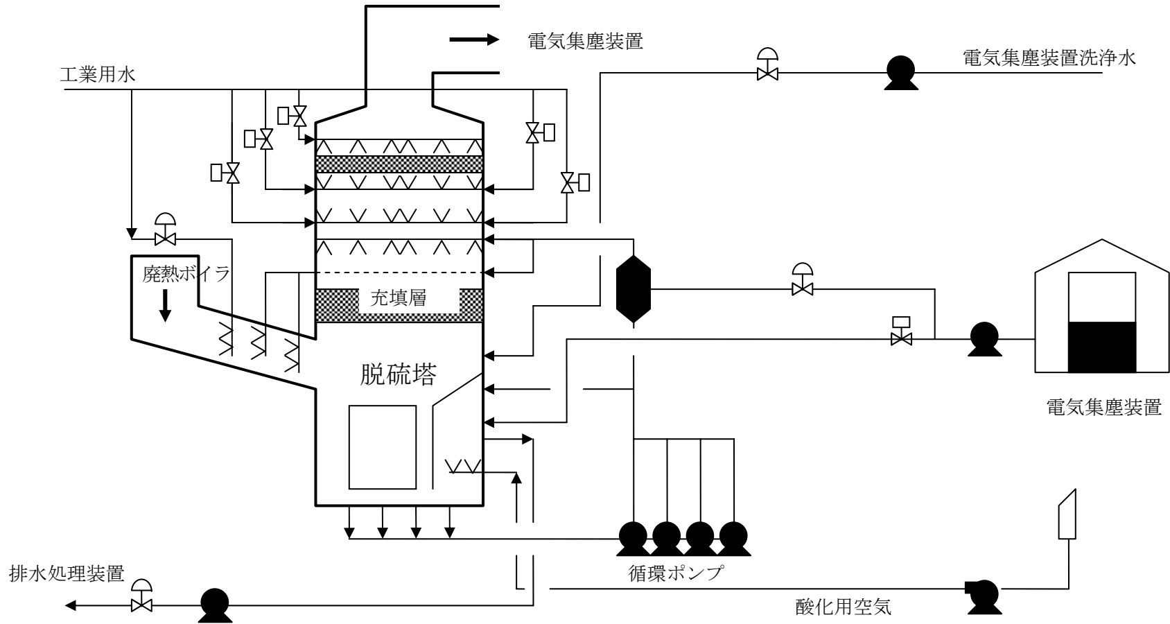
図2 排煙脱硫装置
