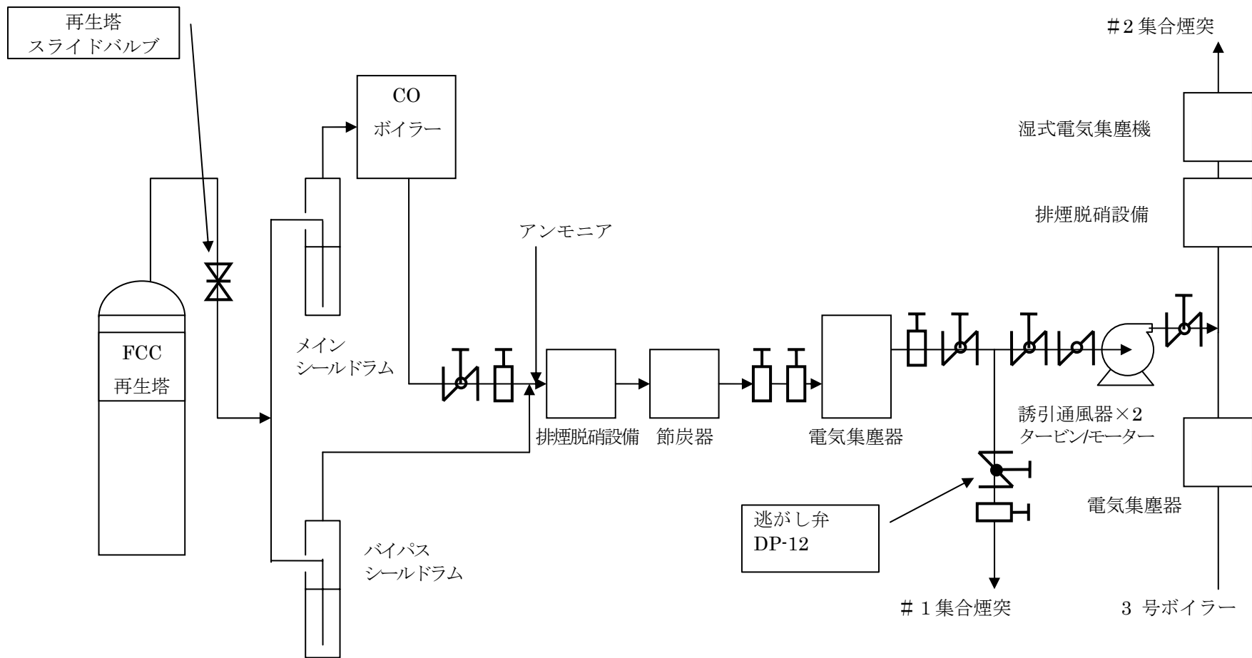
図 1 CO ボイラー廻りのフロー
