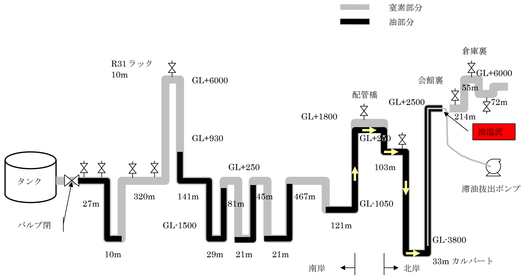
図 配管系統及び管内状態図
