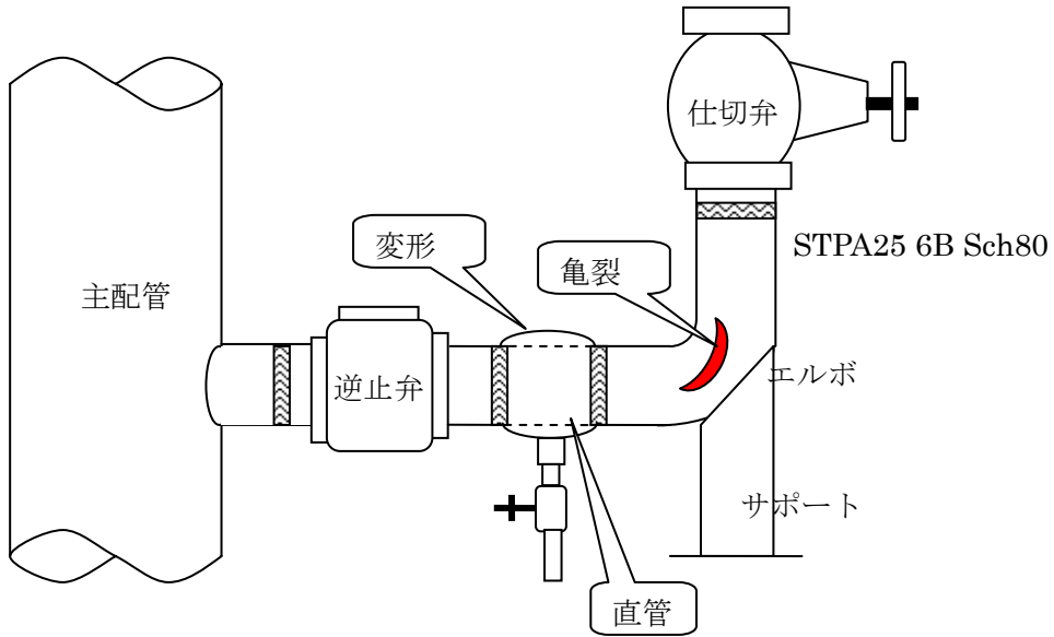
図 2 破裂箇所詳細図
