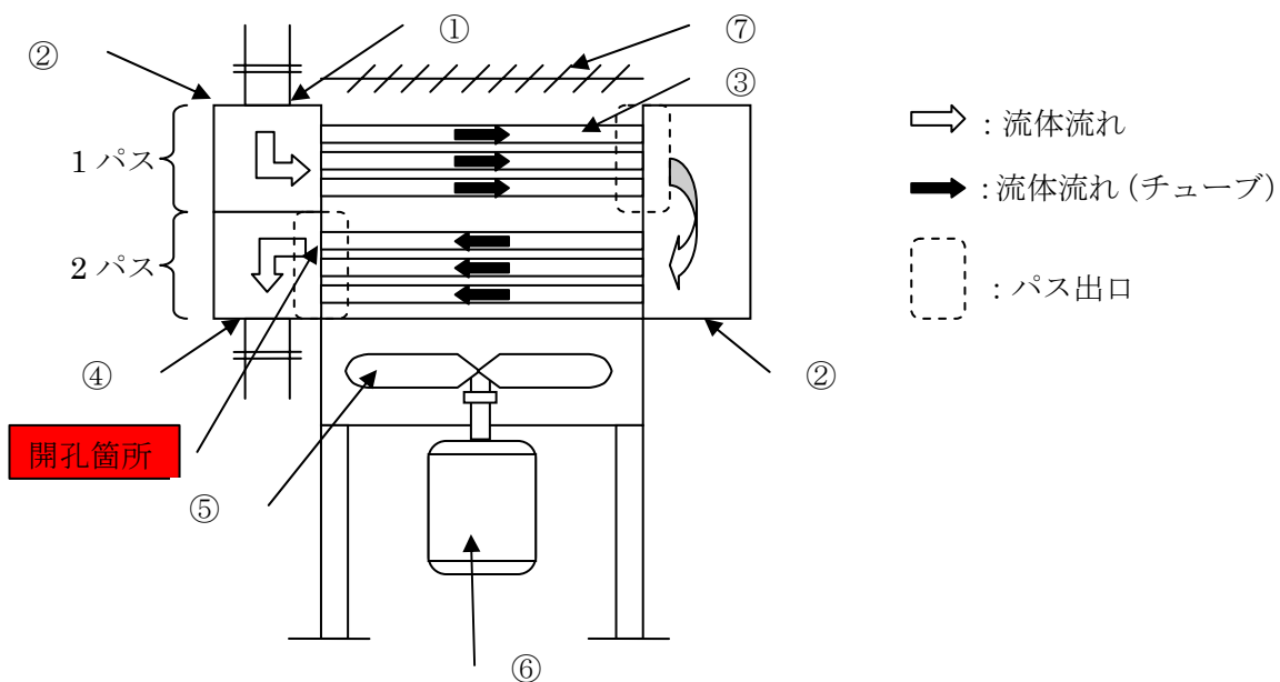
図1 重油直接脱硫装置空気冷却器概略図
